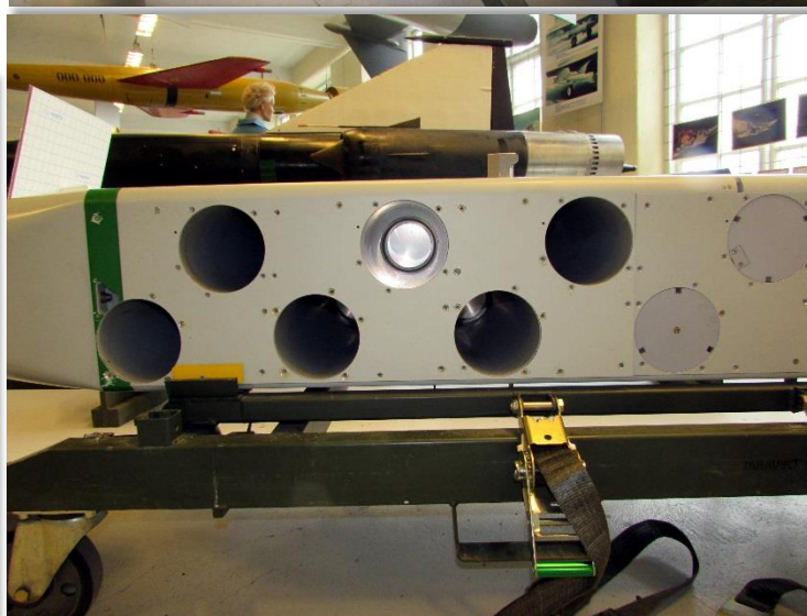
Bombkapseln demonteras.
